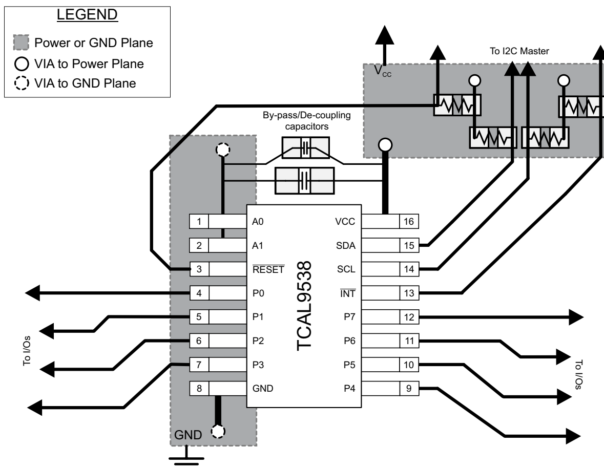
图 8-9. TCAL9538 布局
