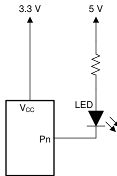
图 8-3. 由较低电压供电的器件
