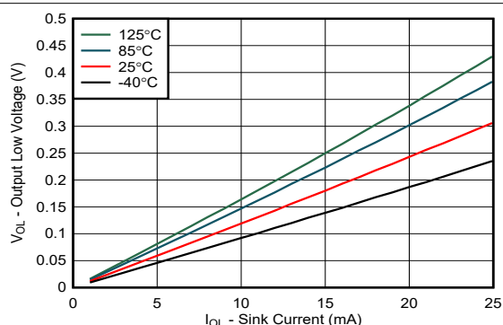
图 5-9. V_{CC} = 3.3\text{V} 时, 不同温度 ( T_A ) 下的 I/O 灌电流与输出低电压间的关系
