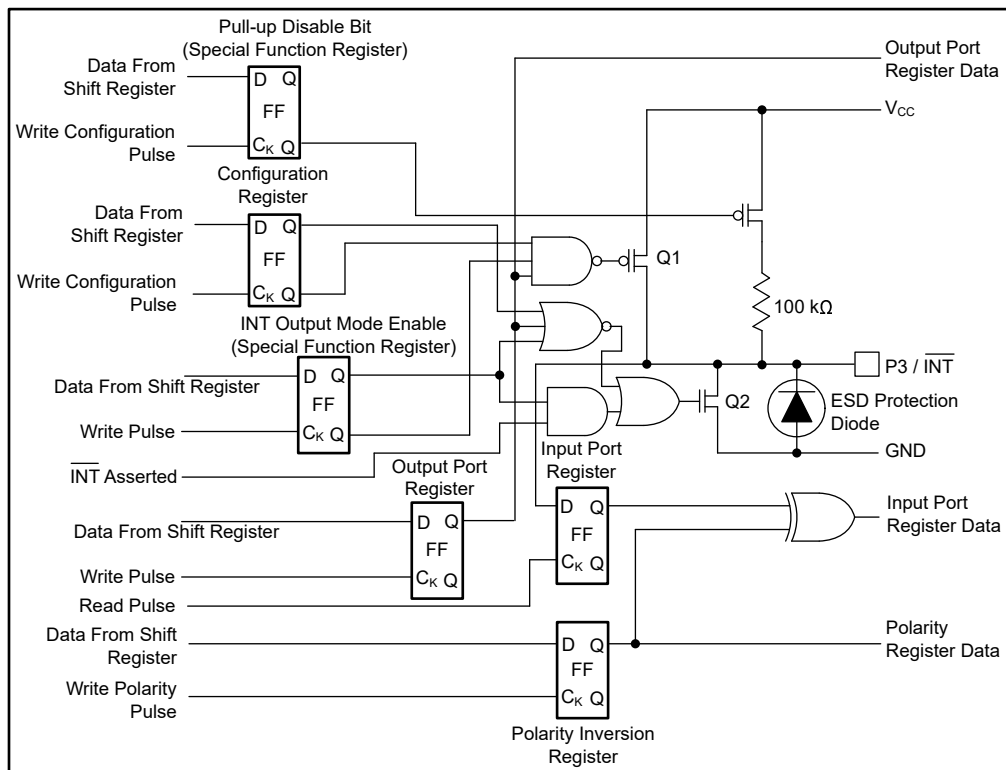
图 7-3. P3/INT 的简化原理图
