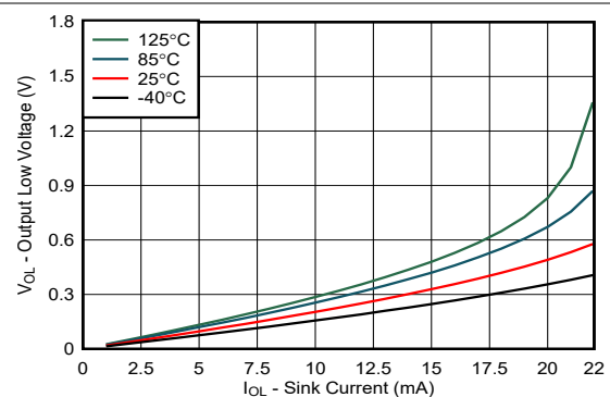
图 5-11. V_{CC} = 1.8\text{V} 时, 不同温度 ( T_A ) 下的 I/O 拉电流与输出高电压间的关系
