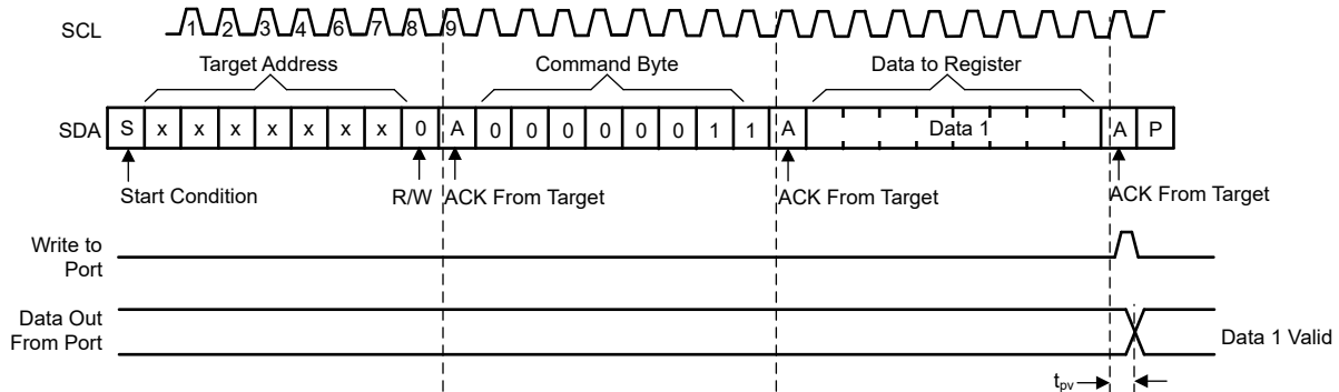
图 7-7. 对输出端口寄存器进行写入
