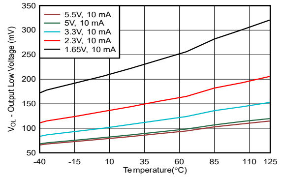
图 5-6. 不同 V_{CC} 下 V_{OL} 与温度间的关系
