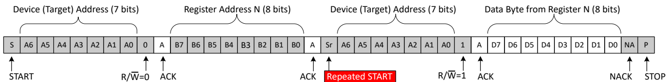
图 7-8. 从寄存器读取
