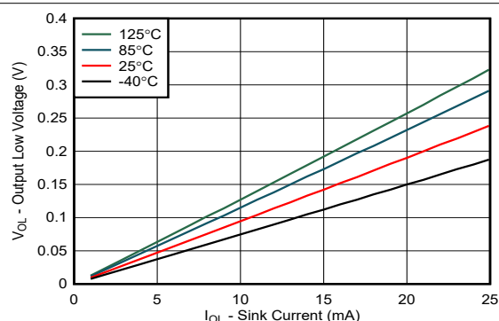
图 5-10. V_{CC} = 5.5\text{V} 时, 不同温度 ( T_A ) 下的 I/O 灌电流与输出低电压间的关系
