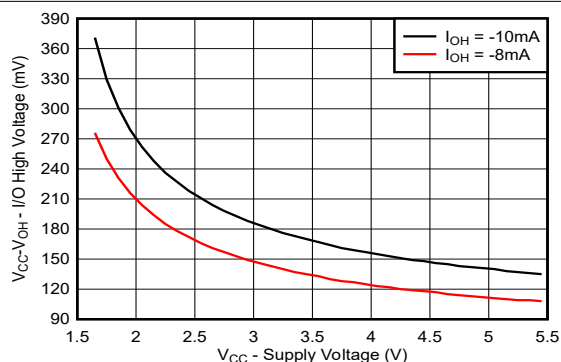
图 5-7. 温度为 25^\circ\text{C} 时, 不同 V_{CC} 下的 V_{CC} - V_{OH} 电压
