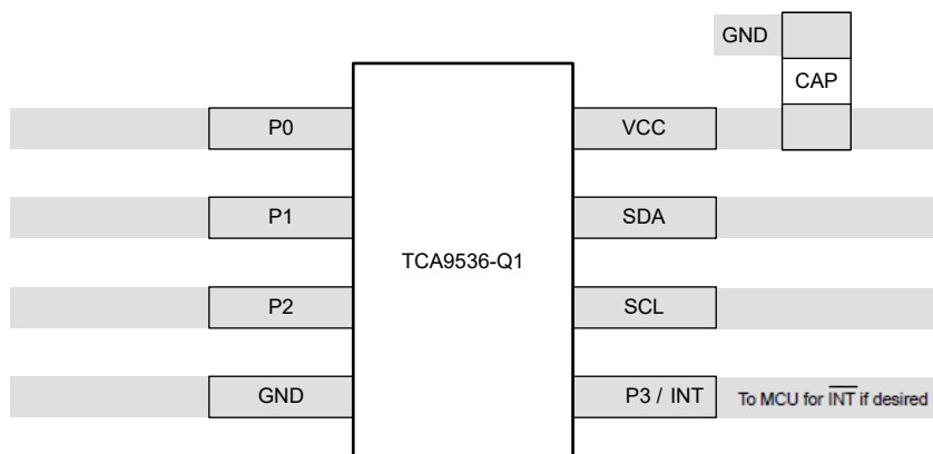
图 10-1. 布局示例 (DGK)
