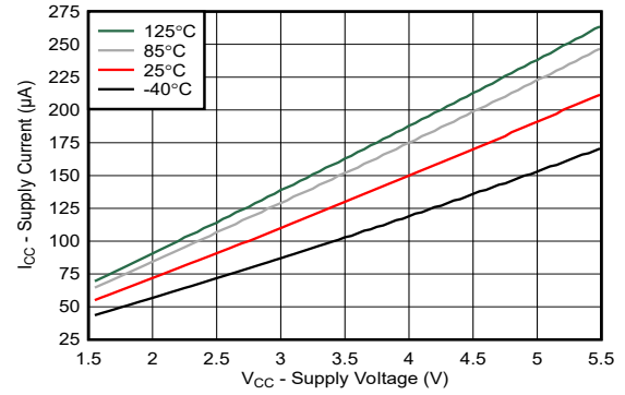
图 5-2. 不同温度 ( T_A ) 下电源电流与电源电压间的关系
