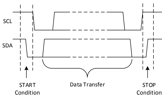
图 7-4. 启动和停止条件的定义
