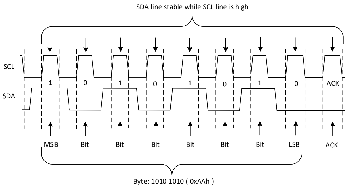
图 7-5. 位传输
