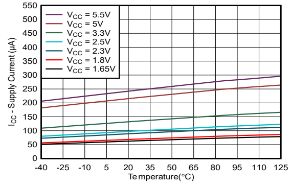
图 5-4. 不同电源电压 ( V_{CC} ) 下电源电流与温度间的关系
