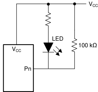
图 8-2. 与 LED 并联的高阻值电阻器
