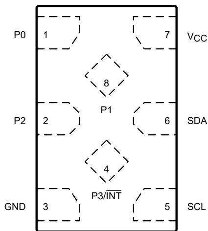
图 4-1. DTM 封装，8 引脚 X2SON，顶视图
