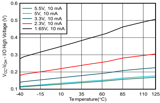
图 5-5. 不同 V_{CC} 下 V_{CC} - V_{OH} 电压与温度间的关系
