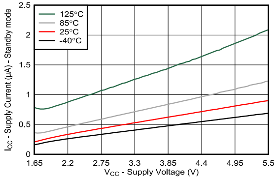
图 5-1. 不同温度 ( T_A ) 下电源电流 (待机) 与电源电压间的关系
