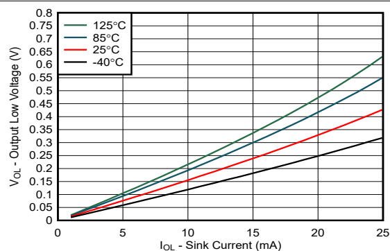
图 5-8. V_{CC} = 2.3\text{V} 时, 不同温度 ( T_A ) 下的 I/O 灌电流与输出低电压间的关系
