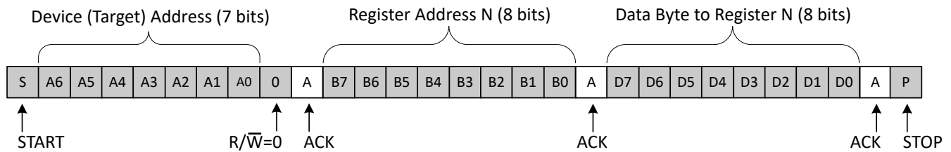
图 7-6. 向寄存器写入
