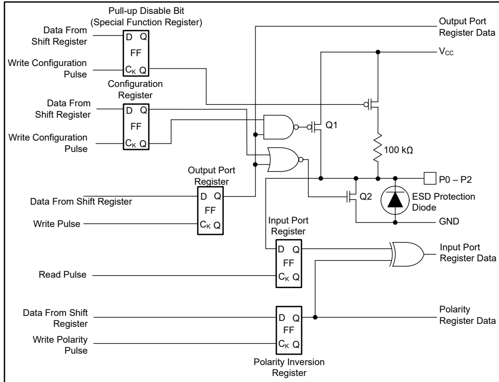
图 7-2. P0 至 P2 的简化原理图
