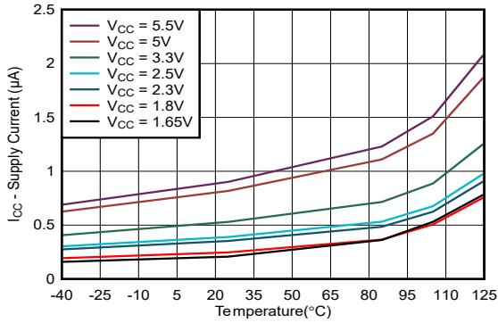
图 5-3. 不同电源电压 ( V_{CC} ) 下待机电源电流与温度间的关系
