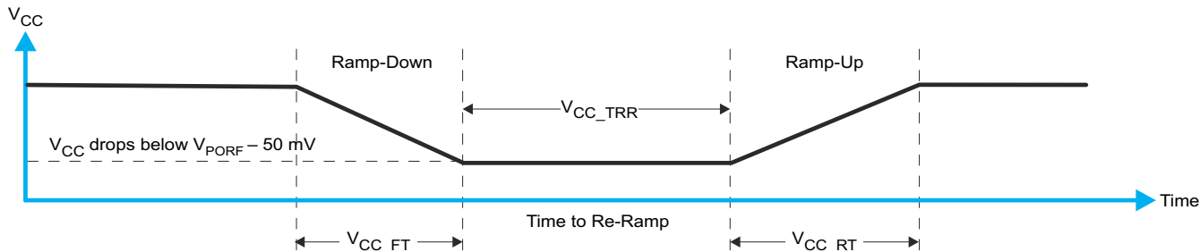
图 9-1. V_{CC} 被降低至低于 POR 阈值，然后重新上升至 V_{CC}
