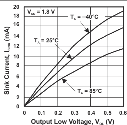
图 6-4. I/O Sink Current vs Output Low Voltage
