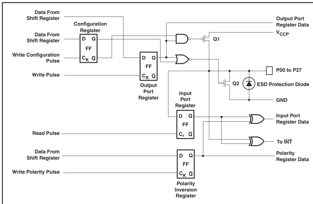
图 8-1. Positive Logic
