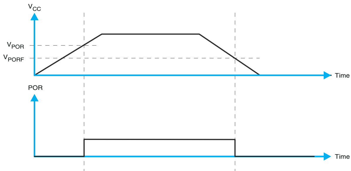
图 9-7. V_{POR}
