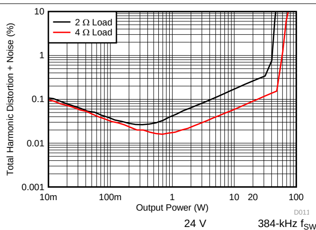
图 10. THD+N vs Power
