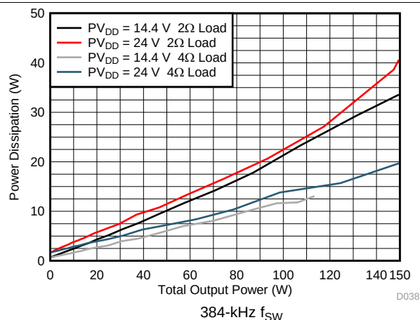
图 33. Power Dissipation vs Output Power
