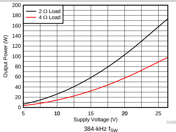
图 31. Output Power vs Voltage
