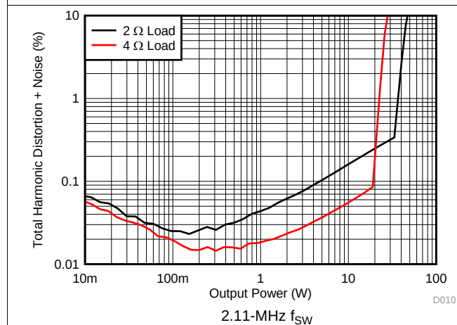
图 9. THD+N vs Power
