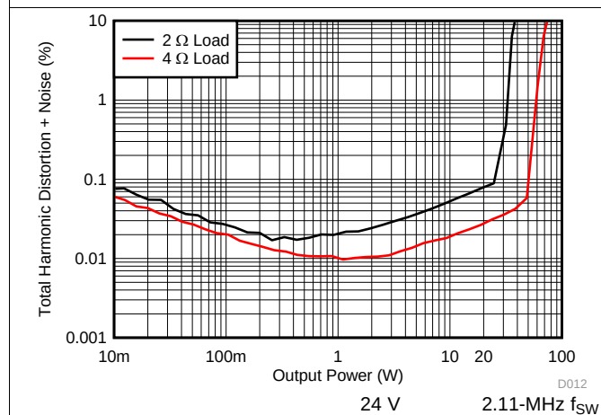
图 11. THD+N vs Power
