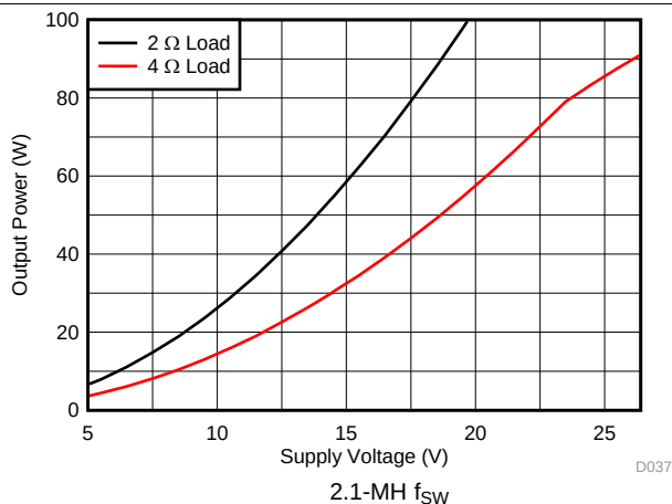
图 32. Output Power vs Voltage
