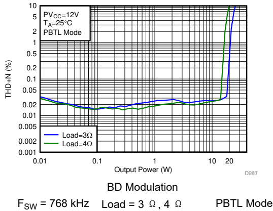
图 7-70. THD+N vs Output Power-PBTL
