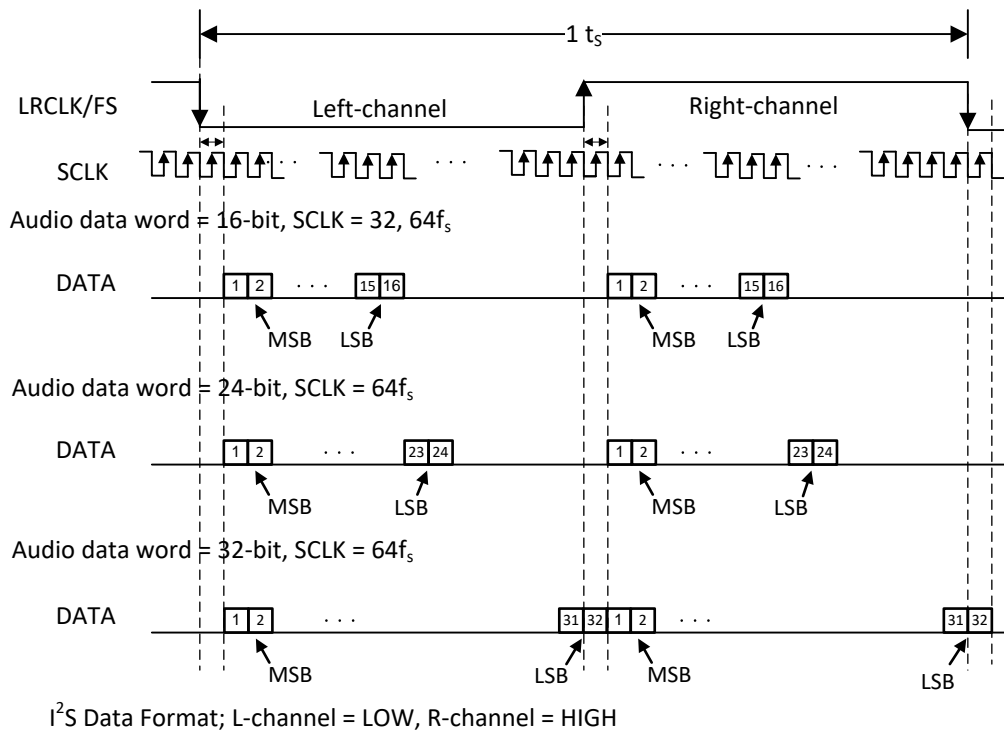
图 68. I²S Audio Data Format
