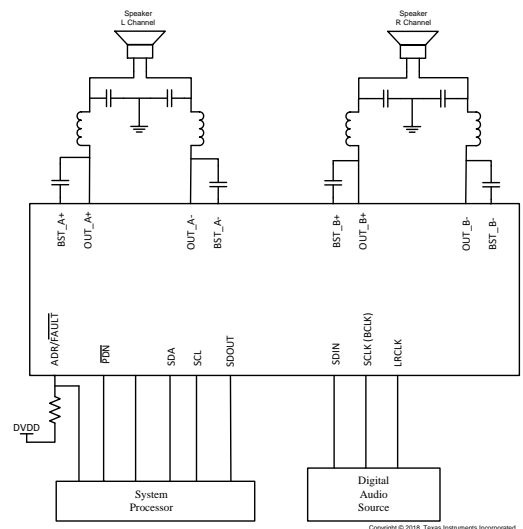
简化方框图
