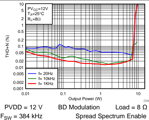
图 37. THD+N vs Output Power
