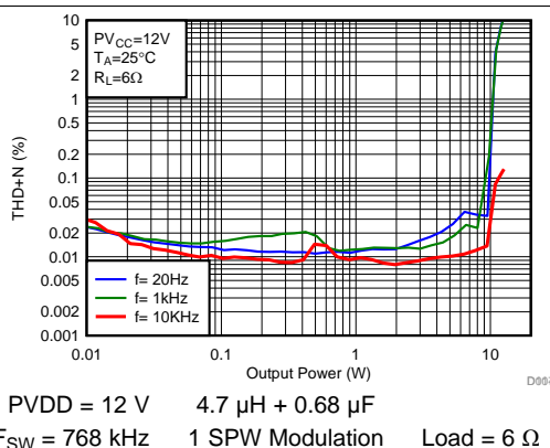
图 118. THD+N vs Output Power
