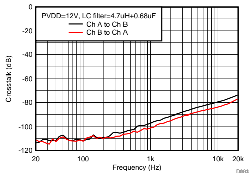
图 27. Crosstalk
