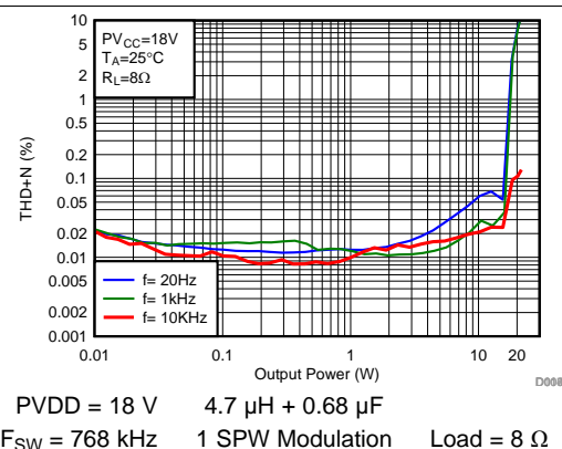
图 119. THD+N vs Output Power
