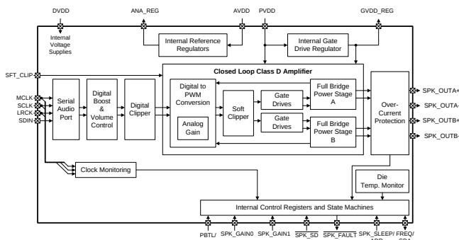
功能方框图
