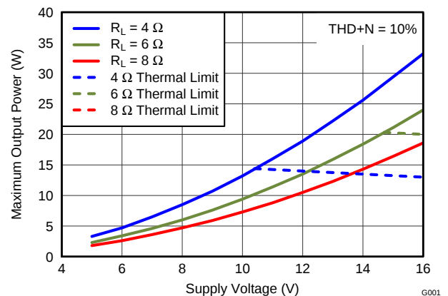
输出功率与 PVDD 间的关系
