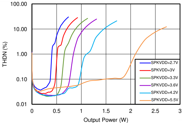
图 9-3. 总谐波失真 + 噪声与 4 \Omega 扬声器功率间的关系
