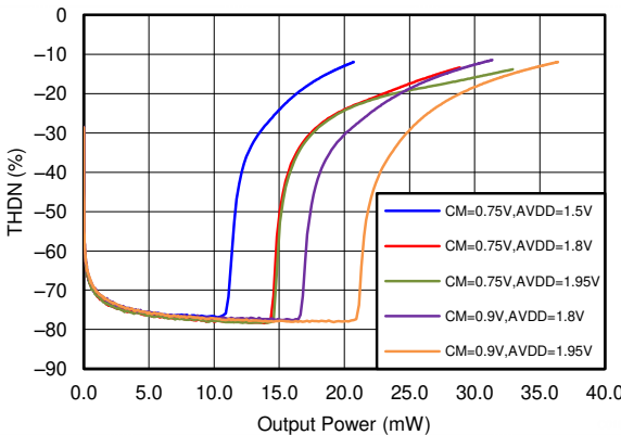
图 9-2. 总谐波失真 + 噪声与 4 \Omega 扬声器功率间的关系
