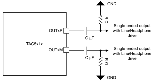
图 6-17. 立体声单端输出连接 (OUT1x_CFG[2:0] = 3'b001)
