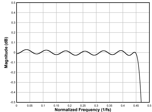
图 6-27. 线性相位内插滤波器通带纹波
