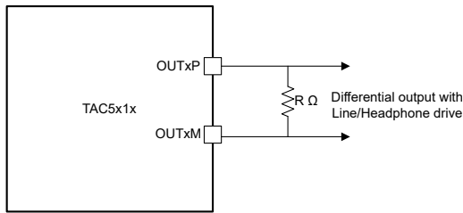
图 6-14. 差分输出连接 (OUT1x_CFG[2:0] = 3'b000)
