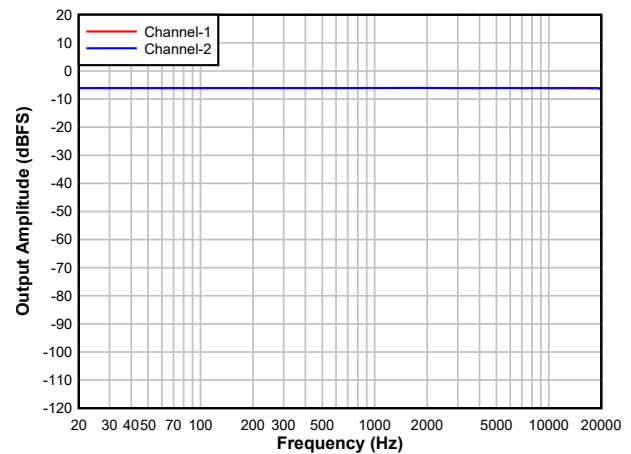
图 6-27. DAC 频率响应
