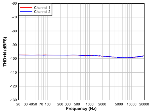
交流耦合单端线路输入 (-60dBFS)
