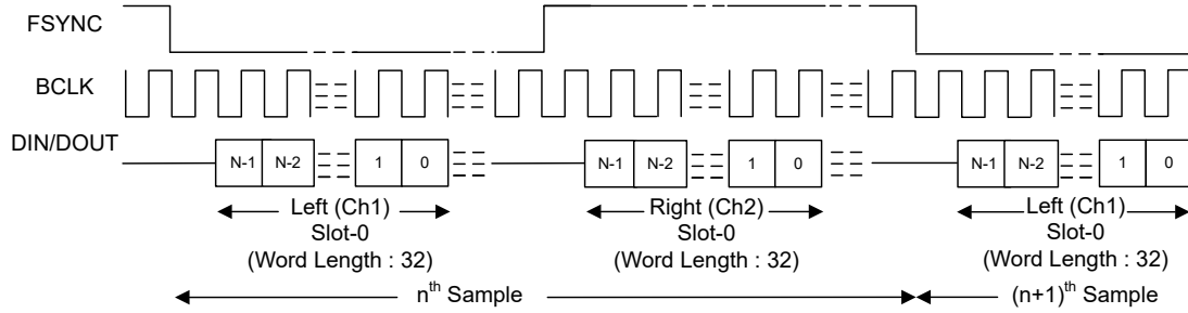
图 7-3. 目标模式下的 I 2 S 模式协议时序 ( MD0 对地短路 )
