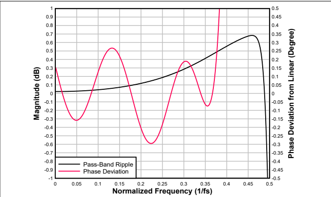
图 7-32. 低延迟抽取滤波器通带纹波和相位偏差
