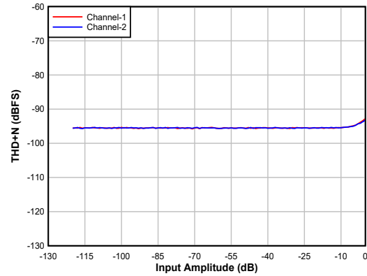
交流耦合单端线路输入
