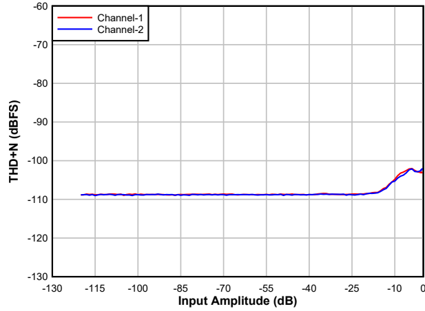
图 6-14. DAC THD + N 级别与输入间的关系
