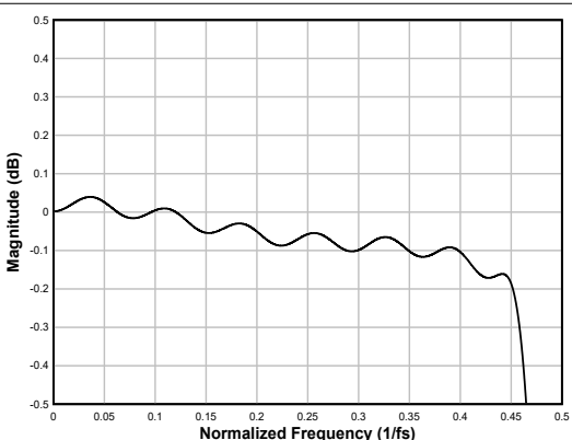
图 7-51. 线性相位内插滤波器通带纹波
