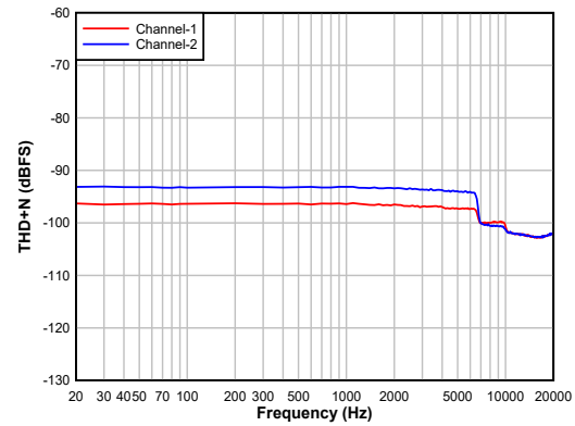
交流耦合差分线路输入 (-1dBFS)
