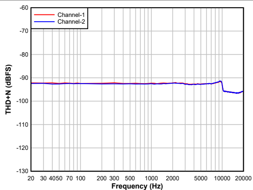
图 6-8. ADC THD+N 与频率间的关系
