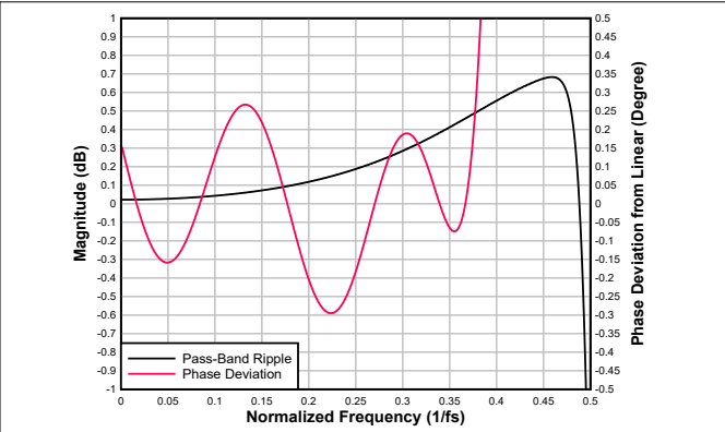
图 7-30. 低延迟抽取滤波器通带纹波和相位偏差
