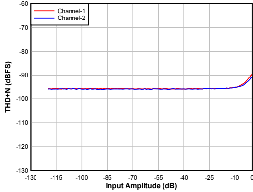
交流耦合差分线路输入， AVDD=1.8\text{V}
