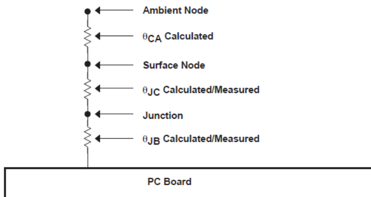
图 7-2. Thermal Resistance
