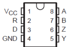
图 4-1. D or P Package (Top View)
