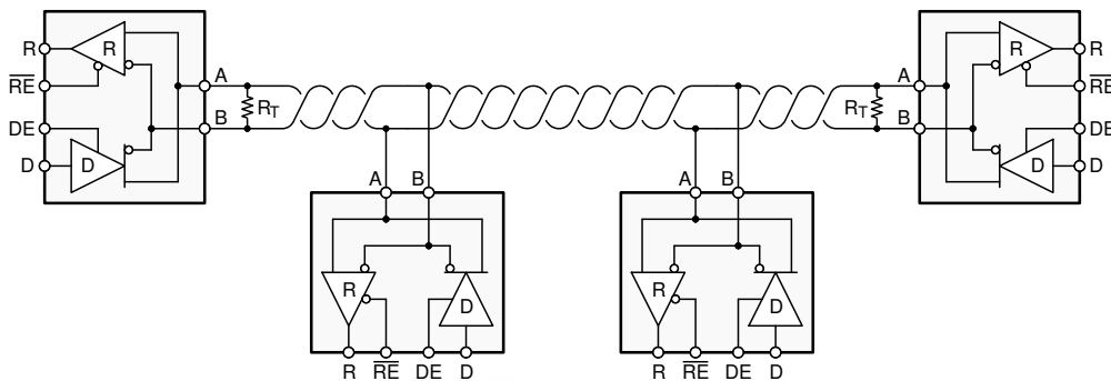
典型应用图
