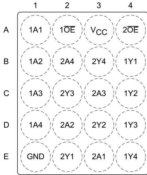
Not to scale 图 4-1. ZQN 封装 20 引脚 BGA 顶视图
