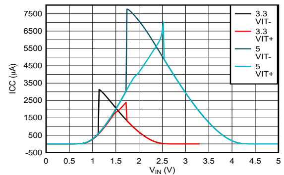
图 5-2. 电源电流与输入电源电压 (3.3V 至 5.0V) 间的关系
