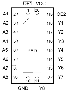
图 4-1. SN74LV8T9541 RKS 封装 (顶视图)
