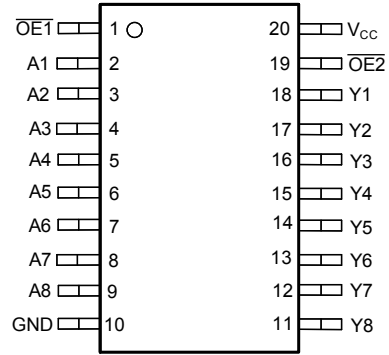
图 4-2. SN74LV8T9541 PW、DGS 封装 (顶视图)
