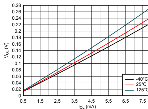
图 5-8. 低电平状态下输出电压与电流间的关系 (1.8V 电源)
