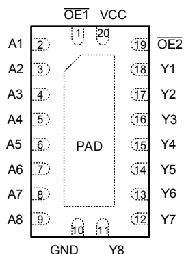
图 4-1. SN74LV8T7541-Q1 RKS 封装 (顶视图)
