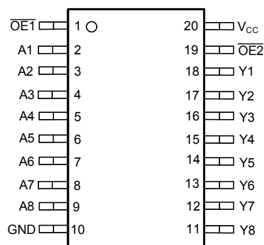
图 4-2. SN74LV8T7541-Q1 PW、DGS 封装 (顶视图)
