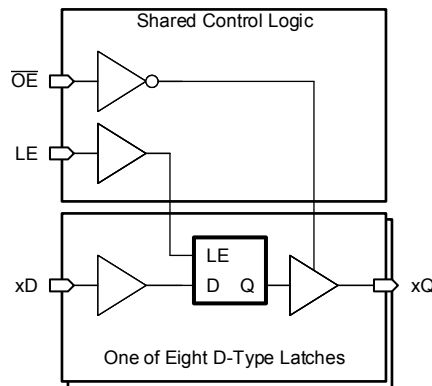
功能方框图
