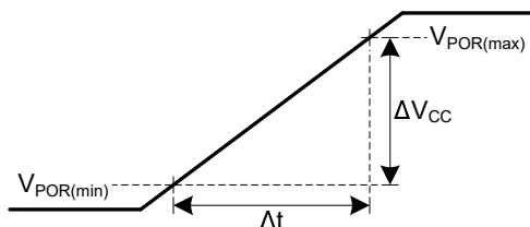
图 7-1. 已知上电状态的电源 ( V_{CC} ) 斜坡特性
