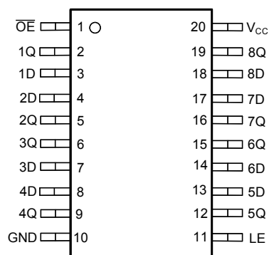
图 4-2. SN74LV8T373 PW、DGS 封装 (顶视图)
