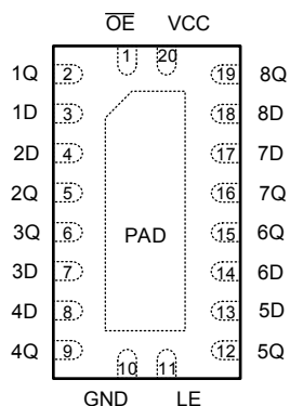
图 4-1. SN74LV8T373 RKS 封装 (顶视图)
