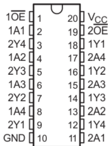
图 4-1. SN74LV8T240 PW 或 DGS 封装；20 引脚 TSSOP 或 VSSOP (顶视图)
