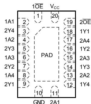
图 4-2. SN74LV8T240 RKS 封装；20 引脚 TSSOP (顶视图)
