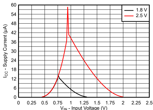
图 6-1. 1.8V 和 2.5V 输入电压电源上的电源电流
