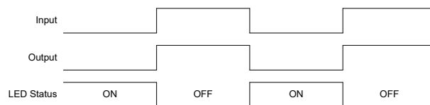
图 9-2. 带 LED 状态的时序图
