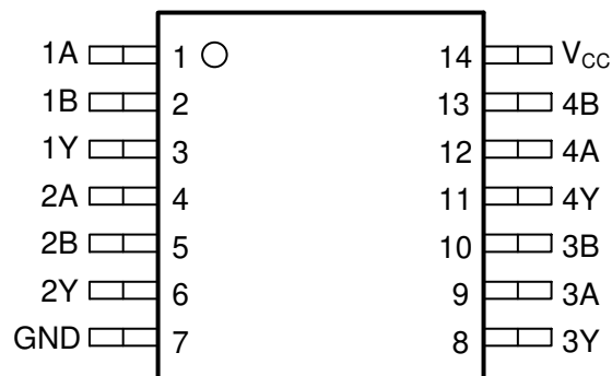
图 5-2. PW 封装，14 引脚 TSSOP (顶视图)
