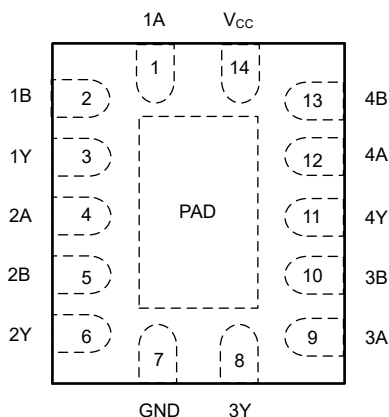
图 5-1. BQA 封装，14 引脚 WQFN (顶视图)
