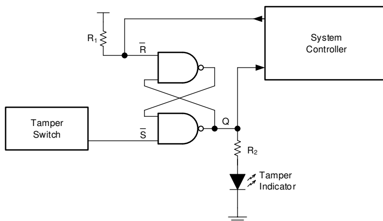
图 10-1. 典型应用框图
