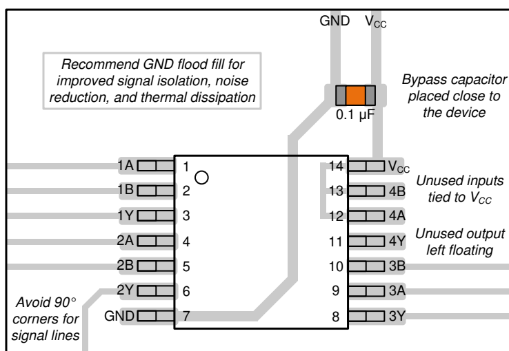
图 12-1. SN74LV4T00 的示例布局
