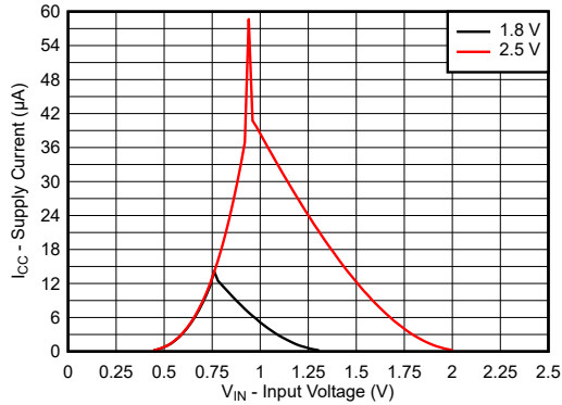
图 7-1. 1.8V 和 2.5V 输入电压电源上的电源电流
