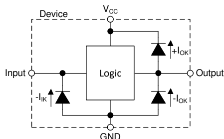
图 9-1. 每个输入和输出的钳位二极管的电气布置
