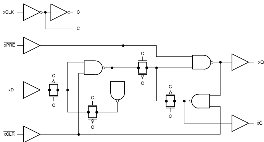
图 8-1. SN74LV2T74 的一个通道的逻辑图 (正逻辑)
