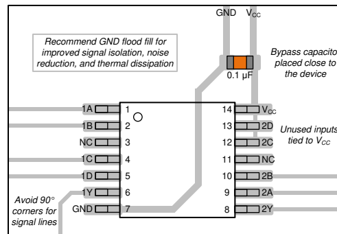
图 11. Example layout for the SN74HCS21-Q1
