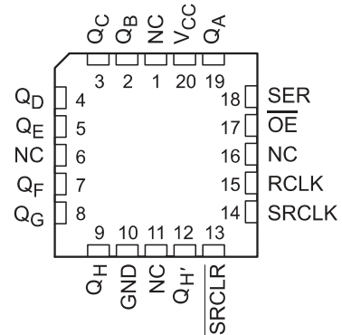
FK 封装 20 引脚 LCCC 顶视图
