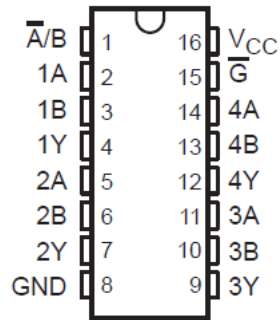
J、D、DB、N、NS 或 PW 封装 16 引脚 CDIP、SOIC、SSOP、PDIP、SO、TSSOP 顶视图
