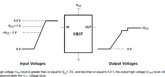
图 7-1. 典型直流电压转换特性
