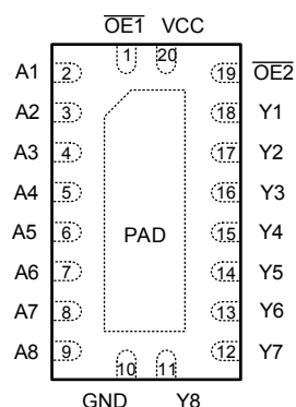
图 4-1. SN74AHCT541-Q1 RKS 封装 (顶视图)
