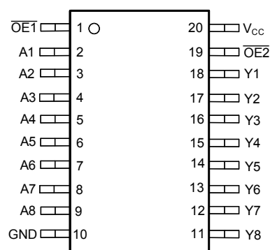
图 4-2. SN74AHCT541-Q1 PW、DGS 封装 (顶视图)
