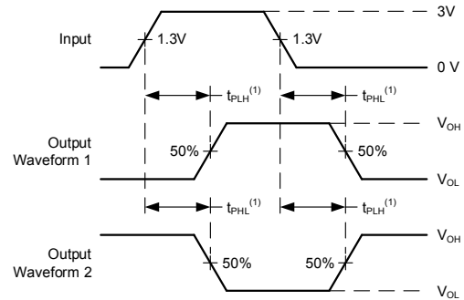
图 6-2. 电压波形传播延迟
