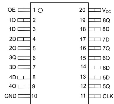
图 4-4. SN74AHCT374 PW、DW、N、DB、DGS 封装 (顶视图)
