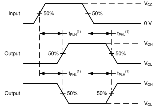
图 6-2. 电压波形传播延迟
