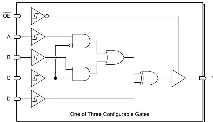
功能方框图
