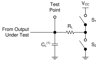
图 6-1. 三态输出的负载电路
