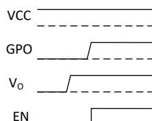
图 8-2. 典型应用时序图
