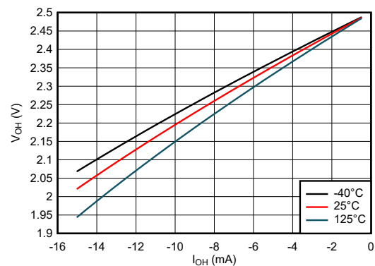
图 6-6. 高电平状态下输出电压与电流间的关系 ; 2.5V 电源
