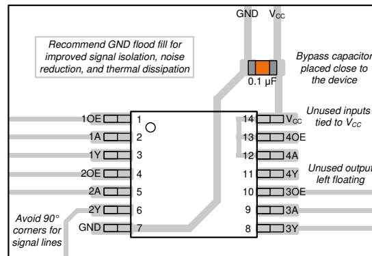
图 9-3. SN74AHC126-Q1 的示例布局
