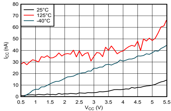
图 6-1. 电源电压两端的电源电流
