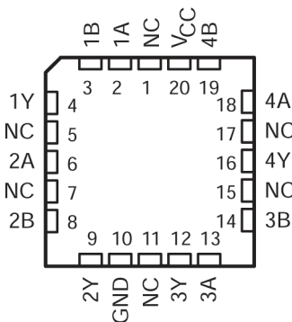
图 3-3. SN54ACT86 FK 封装 (顶视图)
