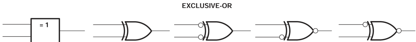
图 6-1. 异或逻辑
