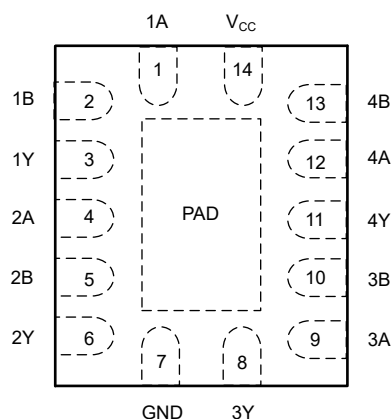
图 3-2. SN74ACT86 BQA 封装 (透明顶视图)
