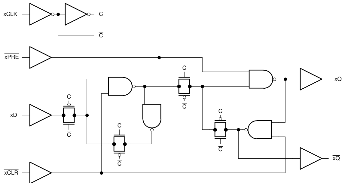
图 7-1. SN74ACT74-Q1 的一个通道的逻辑图 (正逻辑)
