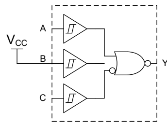
具有 1 个反相输入的双输入或非门
