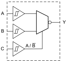
具有反相输出的 2:1 数据选择器
