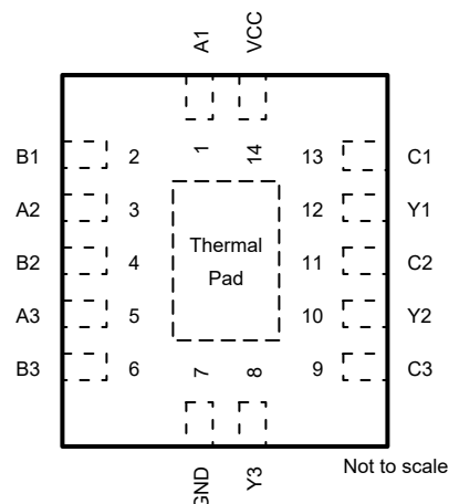
图 4-2. SN74ACT3G98 BQA 封装，14 引脚 WQFN (顶视图)
