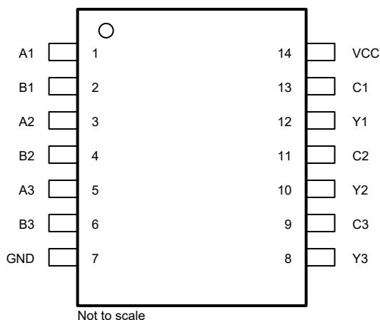
图 4-1. SN74ACT3G98 PW 封装，14 引脚 TSSOP (顶视图)
