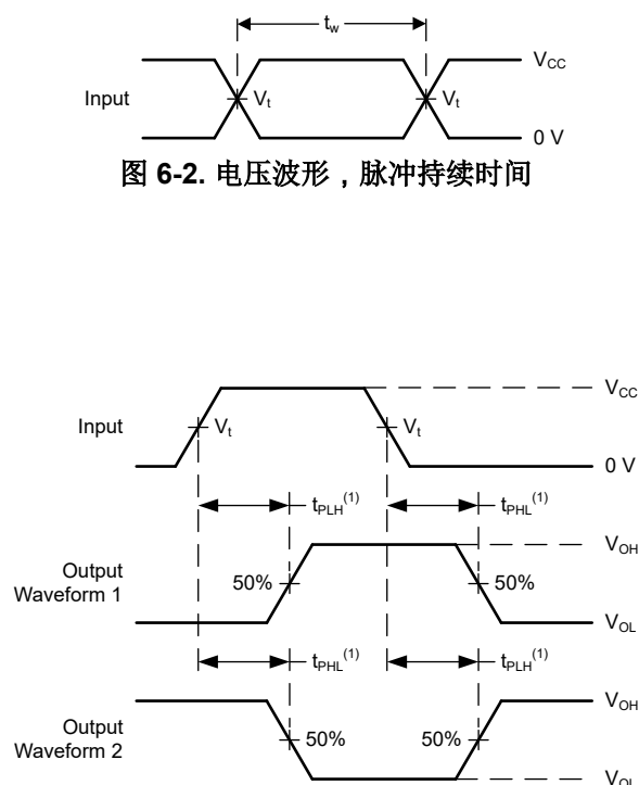
图 6-4. 电压波形传播延迟
