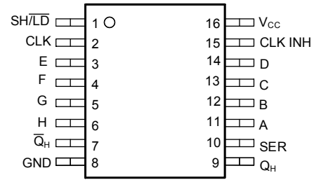
图 4-2. SN74ACT165 PW 封装 (顶视图)
