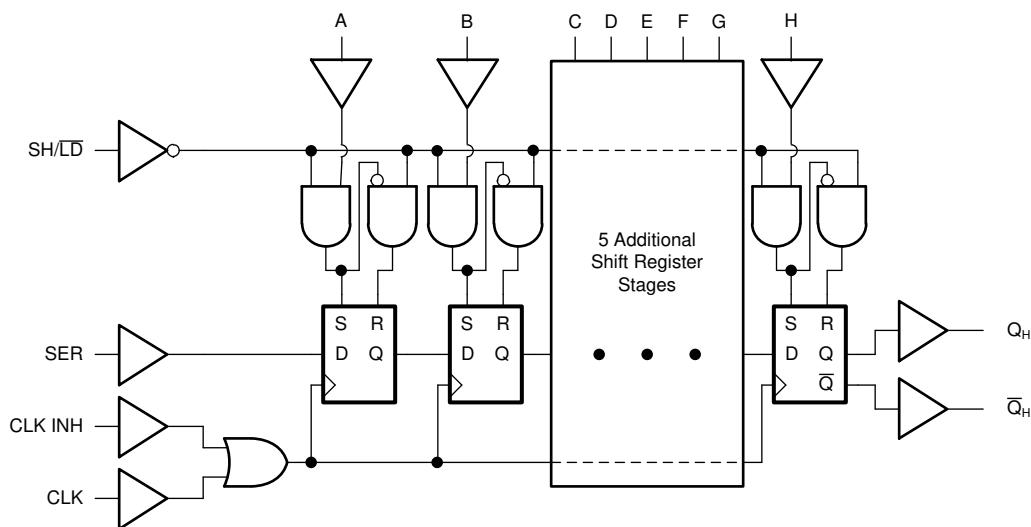
图 7-1. SN74ACT165 的逻辑图 (正逻辑)
