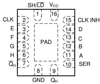
图 4-1. SN74ACT165 BQB 封装 (顶视图)
