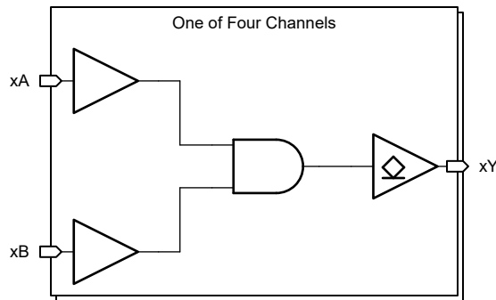
功能方框图
