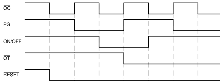
图 8-2. 应用时序图
