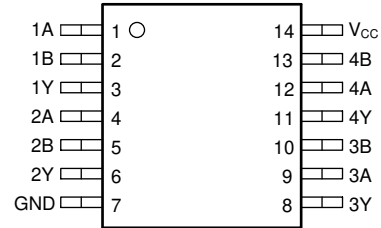
图 4-2. SN74ACT09-Q1、PW 封装 (顶视图)
