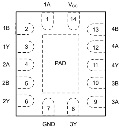
图 4-1. SN74ACT09-Q1 BQA 封装 (顶视图)
