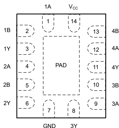
图 3-2. SN74ACT00 BQA 封装 ( 透明顶视图 )
