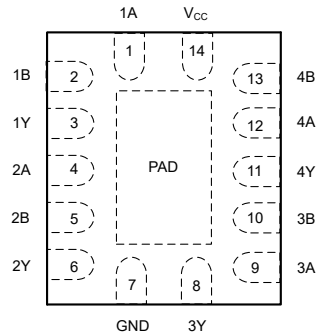
图 3-3. BQA 封装（顶视图）
