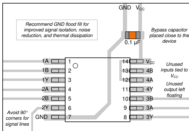
图 7-1. SN74AC86 的示例布局
