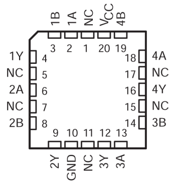
图 3-2. SN54AC86 FK 封装（顶视图）
