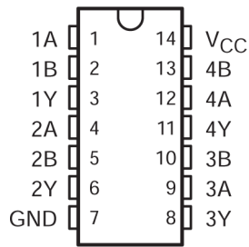
图 3-1. SN54AC86J 或 W 封装；SN74AC86D、DB、N、NS 或 PW 封装（顶视图）
