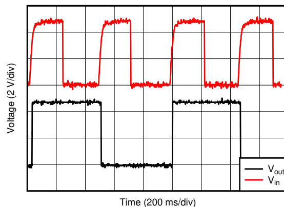
图 8-3. 去抖开关的波形
