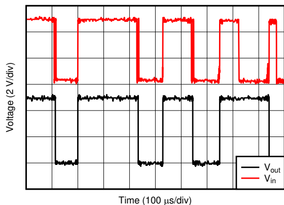
图 8-2. 非去抖开关的波形
