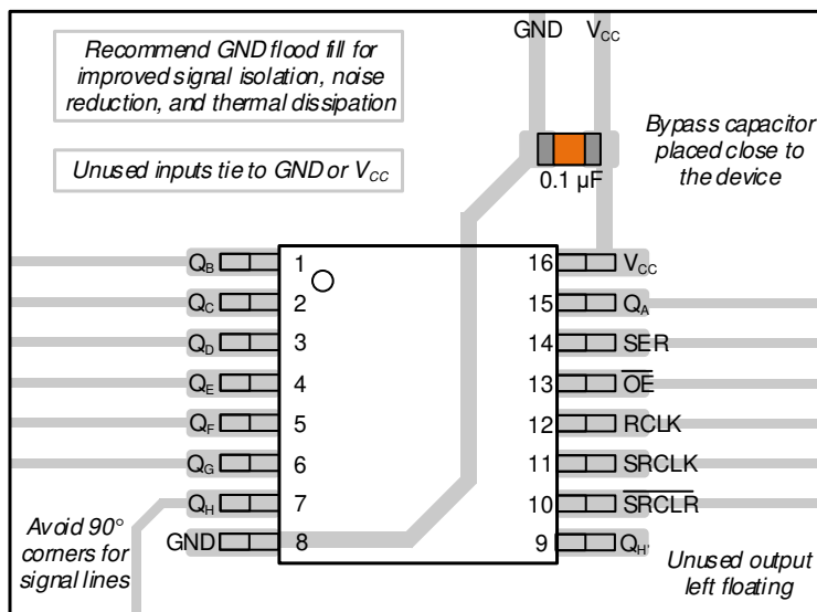
图 8-3. SN74AC595 的示例布局
