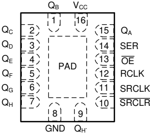
图 4-2. BQB 封装，16 引脚 WQFN (顶视图)
