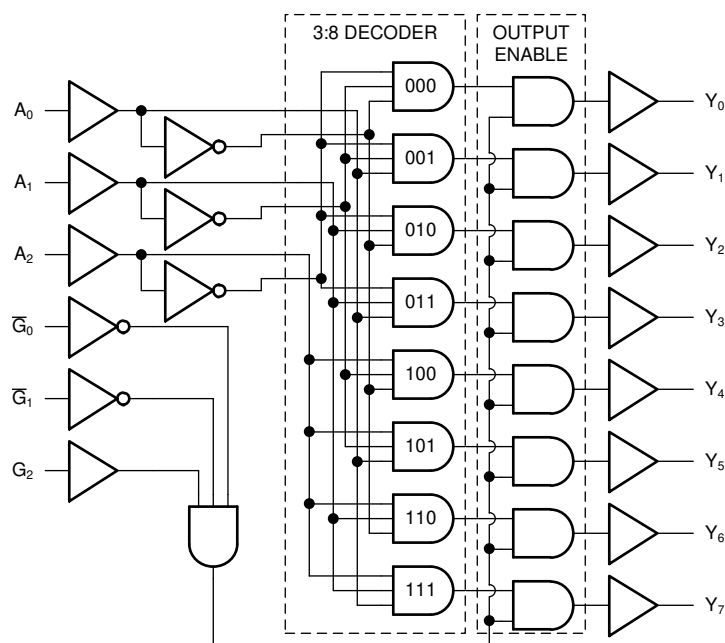
图 7-1. SN74AC238-Q1 的逻辑图 (正逻辑)
