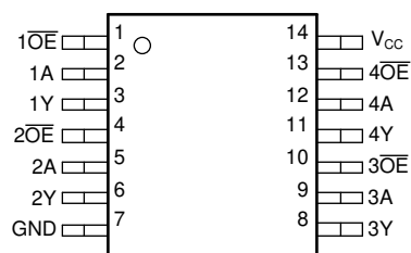
图 4-2. SN74AC125、PW 封装 (顶视图)
