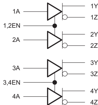
逻辑图（正逻辑）
