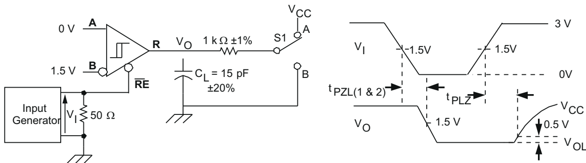
图 7-10. 接收器高电平启用和禁用时间测试电路和电压波形
