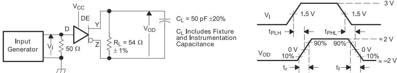
图 7-5. 驱动器开关测试电路和电压波形
