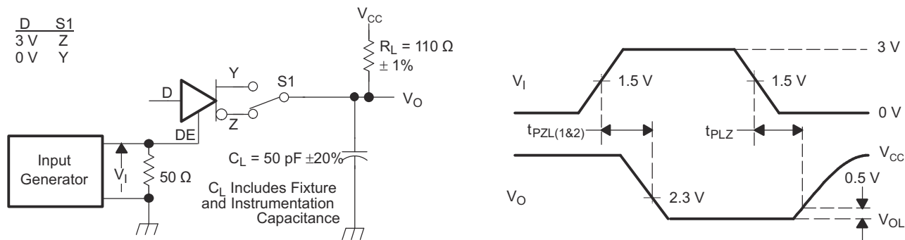
图 7-6. 驱动器高电平输出启用和禁用时间测试电路和电压波形
