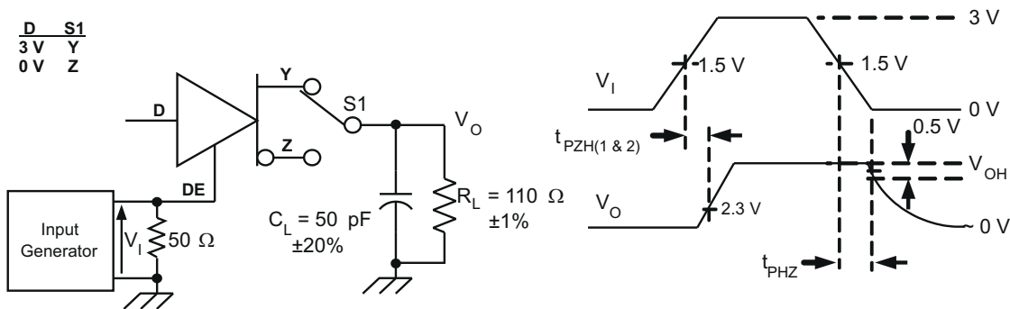
图 7-5. 驱动器开关测试电路和电压波形
