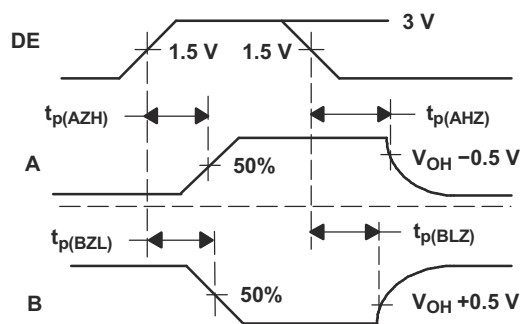
图 7-7. Driver Enable/Disable Test
