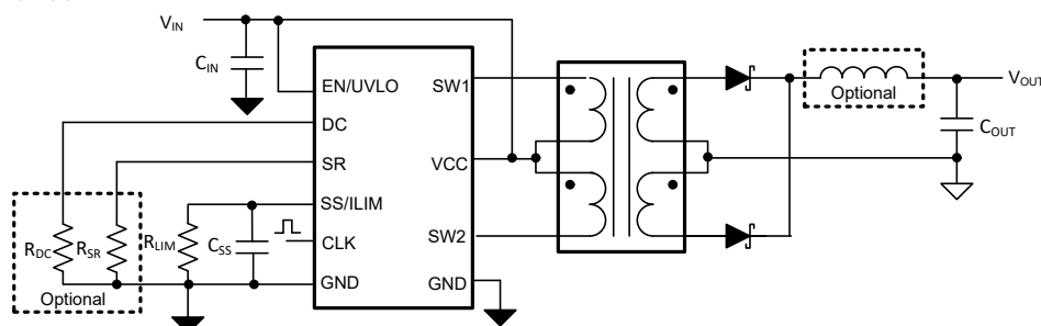
简化原理图
