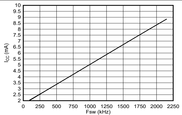
图 6-6. I_{CC} vs Switching Frequency
