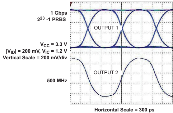
图 9-6. LVDS Output
