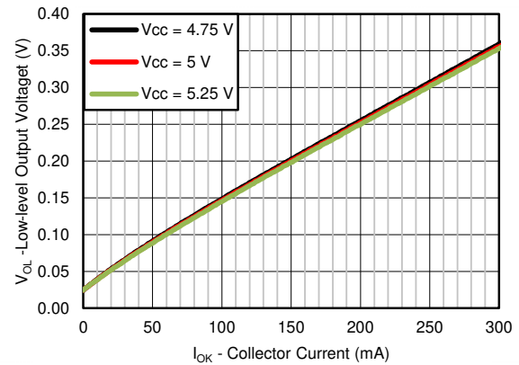
图 9-3. SN75451B 典型低电平输出电压与集电极电流间的关系
