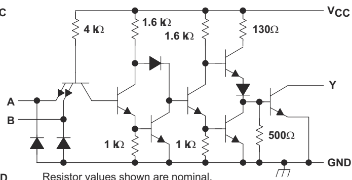
图 8-10. SNx5452B 原理图 (每个驱动器)
