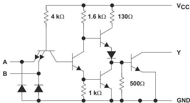
图 8-9. SNx5451B 原理图 (每个驱动器)
