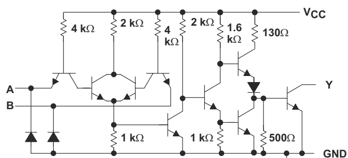
图 8-12. SNx5454B 原理图 (每个驱动器)
