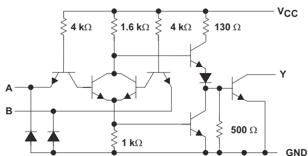
图 8-9. SNx5451B 原理图 (每个驱动器)
