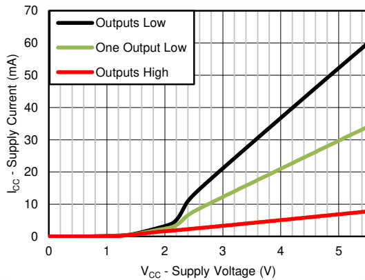
图 9-2. SN75451B 典型电源电流与电源电压间的关系
