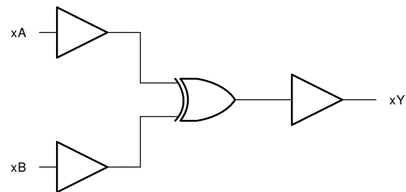
简化逻辑图
